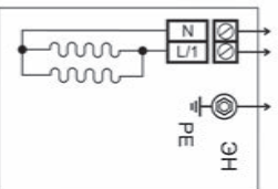
Схема 2. Подключение ЭН «Премьера» с пультом ПУ-01М к сети 220В.
