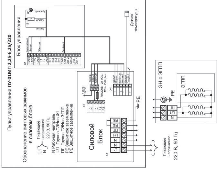
Рис 6. Схема пульта ПУ-01МП 2,25-6,25\220
