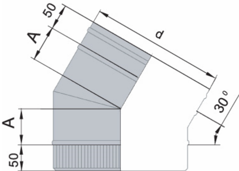
Отвод ОТН 30°
